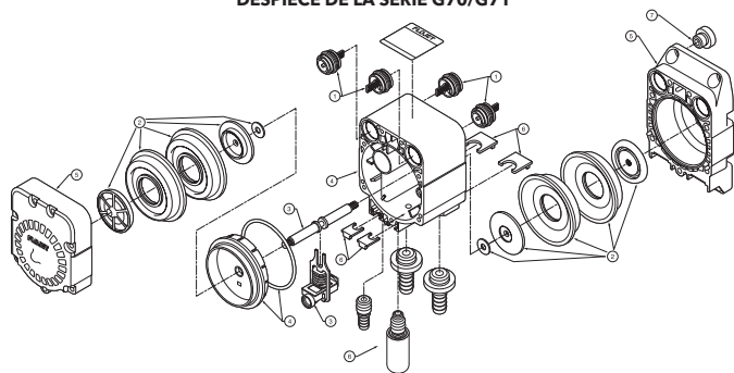
DESPIECE DE LA SERIE G70/G71
